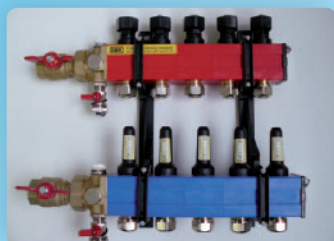
Distribuitor/colector
